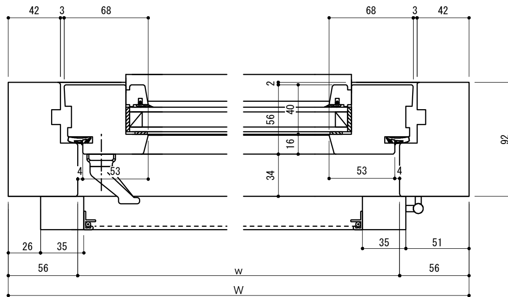
〈よこ断面図〉
