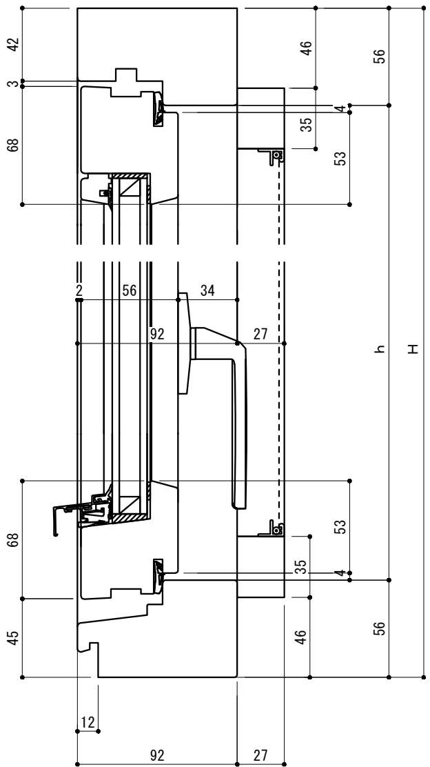
〈たて断面図〉
