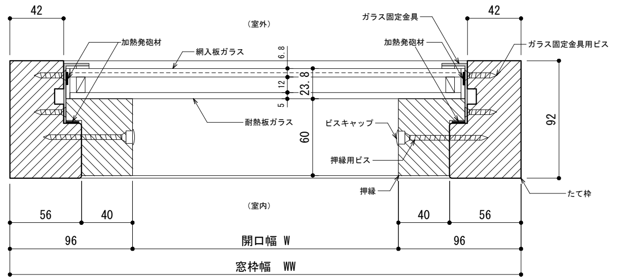
〈よこ断面図〉
