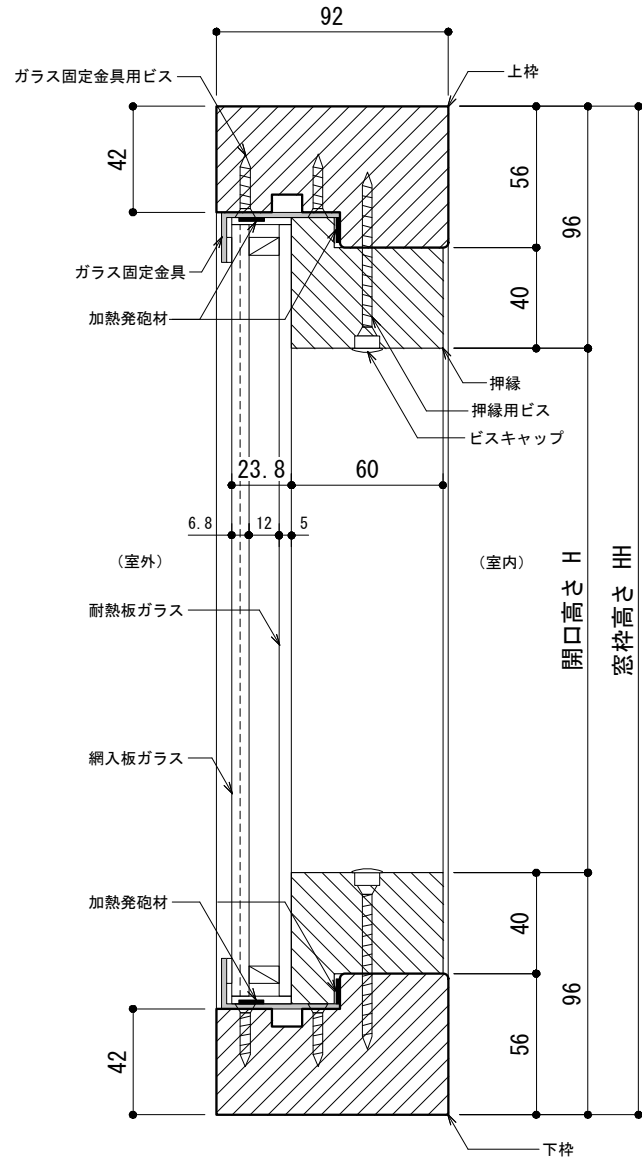
〈たて断面図〉
