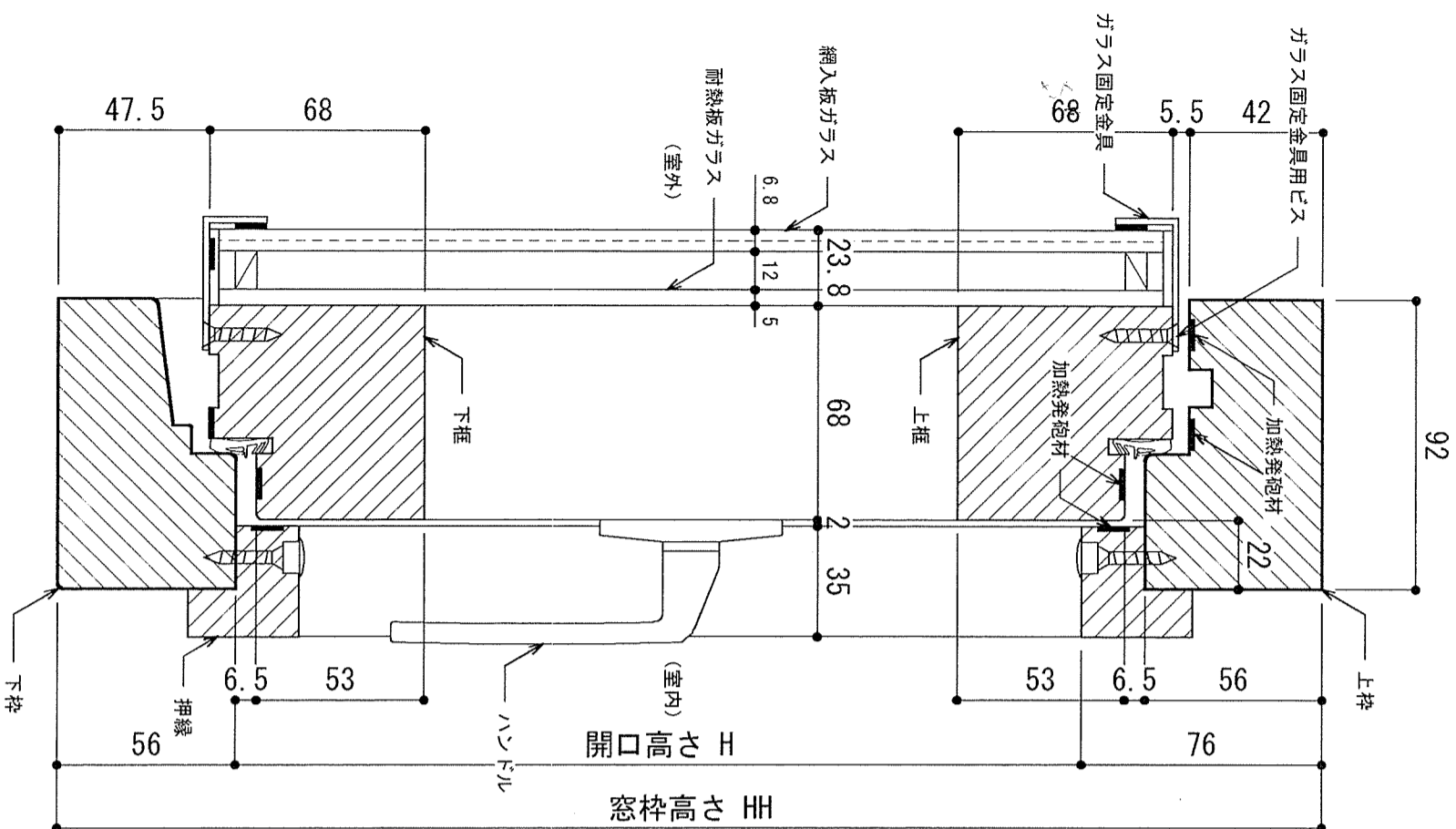
〈たて断面図〉
