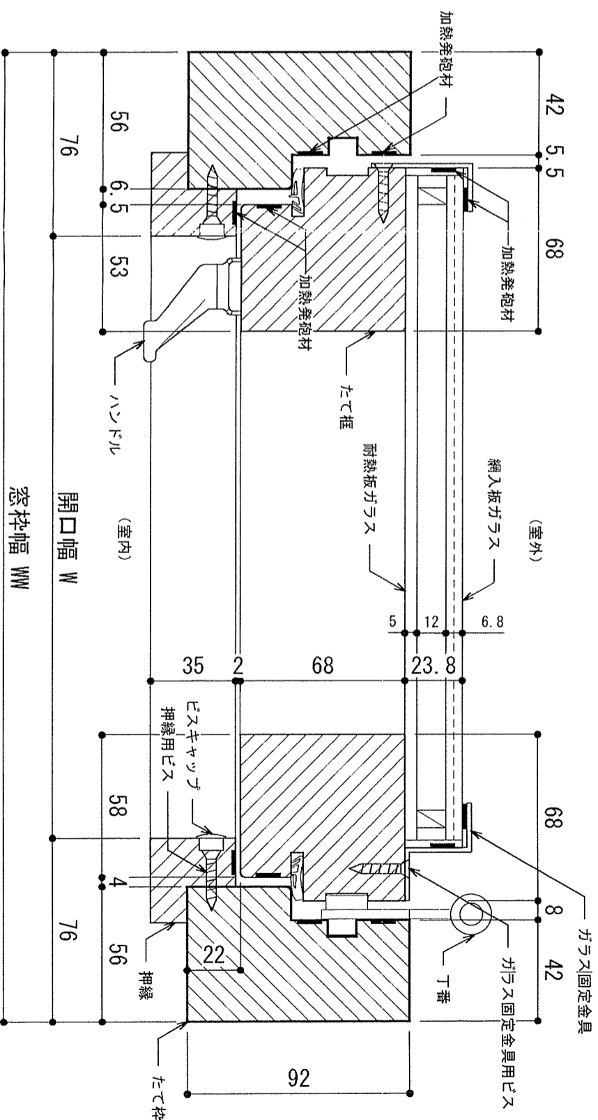
〈よこ断面図〉
