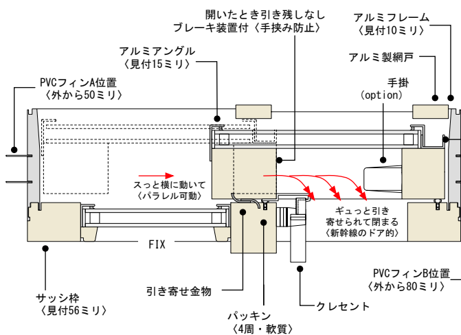
【図9 片引き窓断面】
