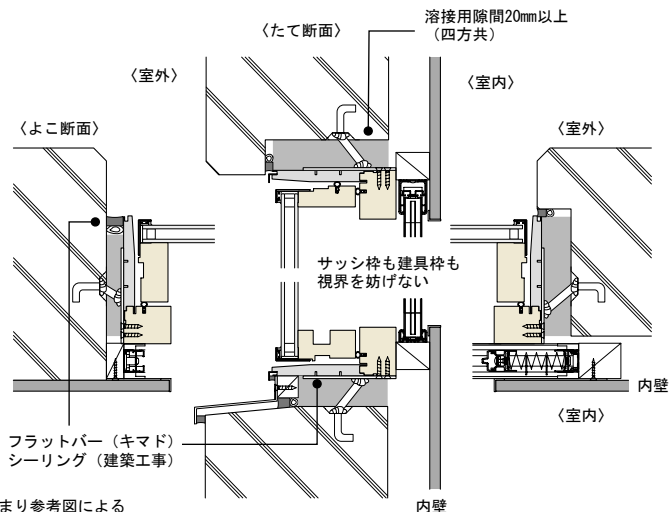
【図18 納まり参考図（突き出し窓、RC）】
