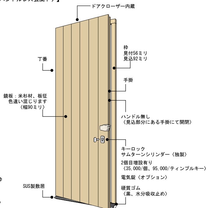
【図12 ハンドルレス玄関ドア】
