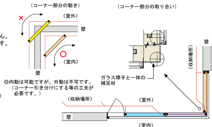
【図26 ドルフィンサッシ参考例 その5 (外開き・コーナータイプ)】
