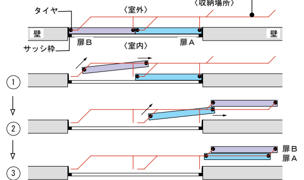
【図25 ドルフィンサッシ動作例 その4 (内開き)】
