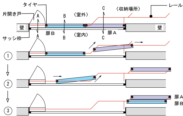
【図23 ドルフィンサッシ参考例 その2 (外開き・並列列動作タイプ)】
