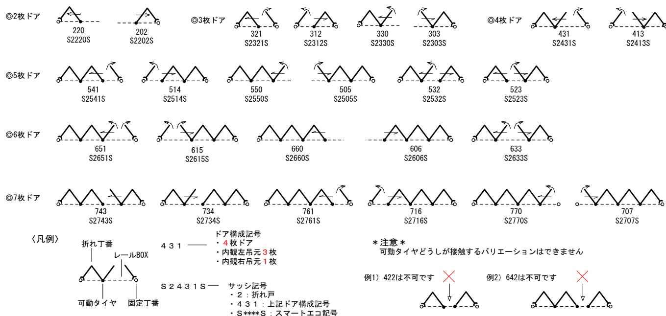
【図16 折れ戸納まり参考図 (330・S2330S)】
