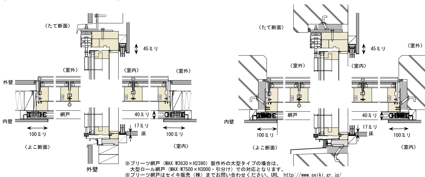
【図16 折れ戸納まり参考図 (330・S2330S)】
