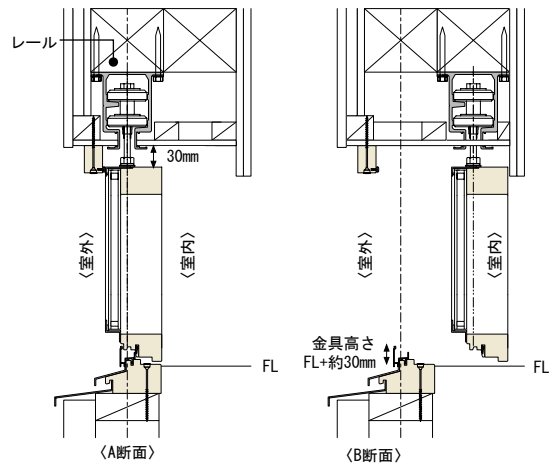
【図26 ドルフィンサッシ参考例 その5 (外開き・コーナータイプ)】
