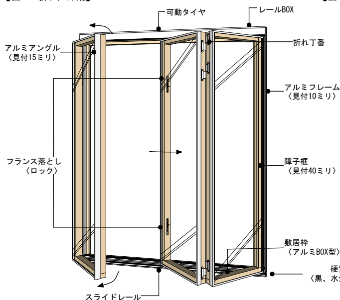
【図13 折れ戸外観】
