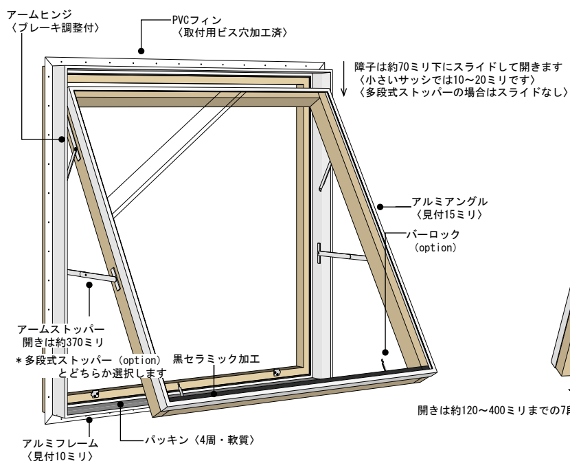
【図4 突き出し窓内観】
