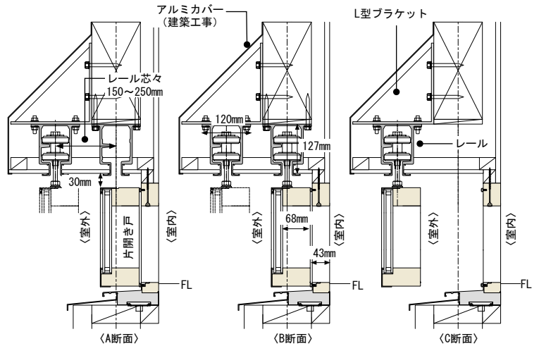
【図24 ドルフィンサッシ参考例 その3 (外開き・90°動作タイプ)】
