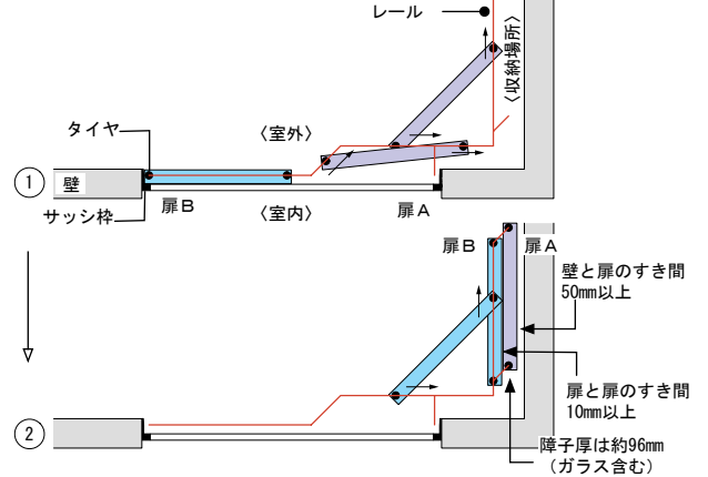
【図24 ドルフィンサッシ参考例 その3 (外開き・90°動作タイプ)】
