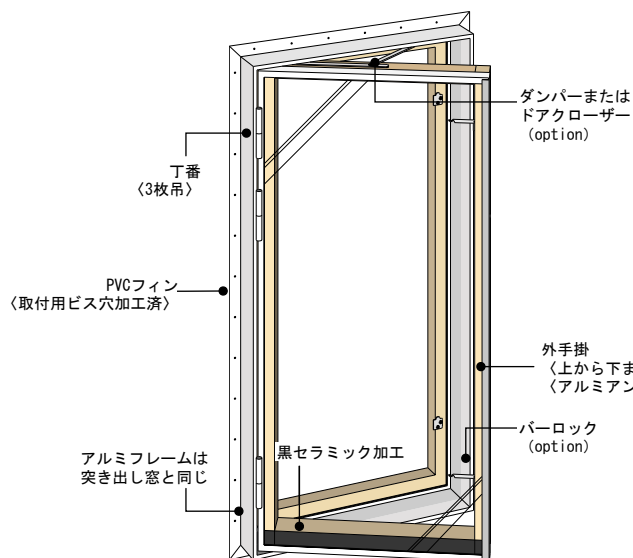
【図7 片開き窓外観・パーロック付】
