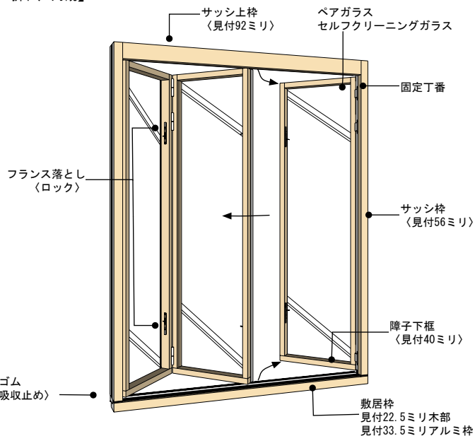
【図14 折れ戸内観】
