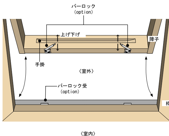
【図5 手掛及びロックシステム1】
