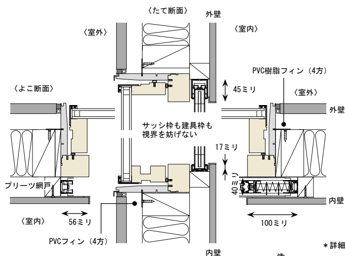
【図19 プリーツ網戸の納まり参考図】
