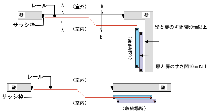
【図25 ドルフィンサッシ動作例 その4 (内開き)】
